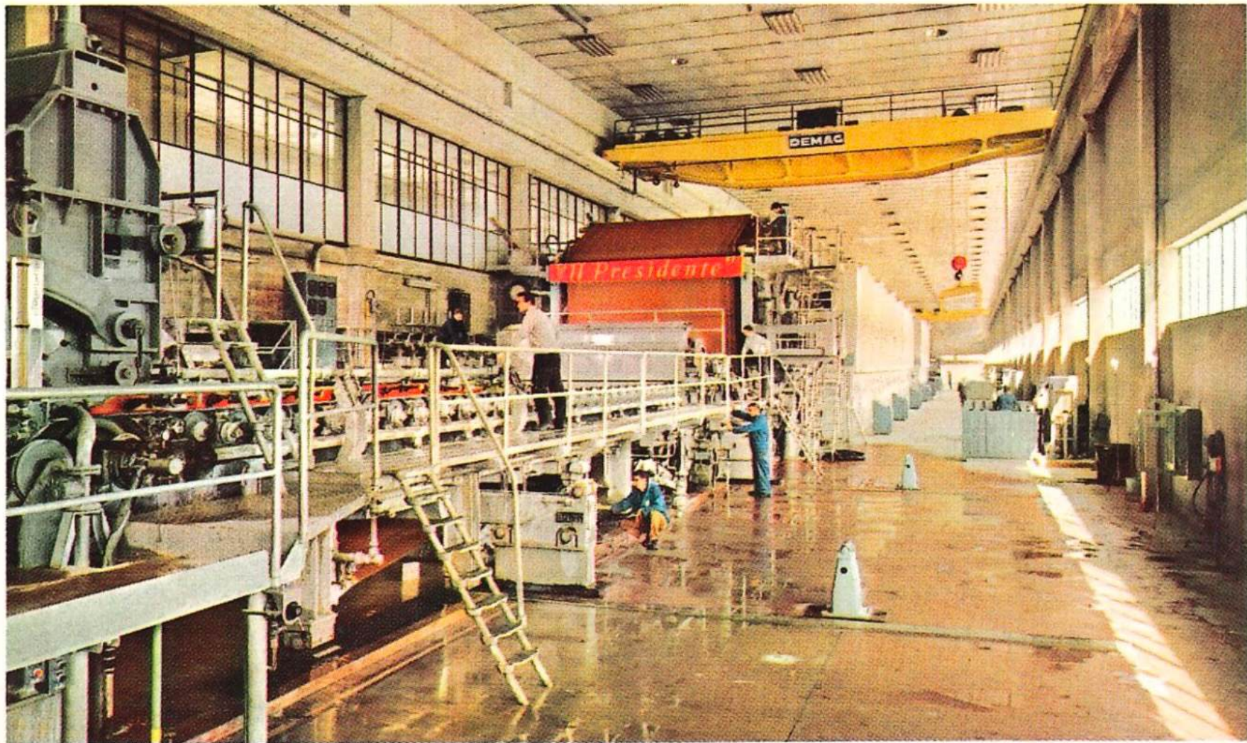
Cartiera di Ascoli: la macchina « continua ».
